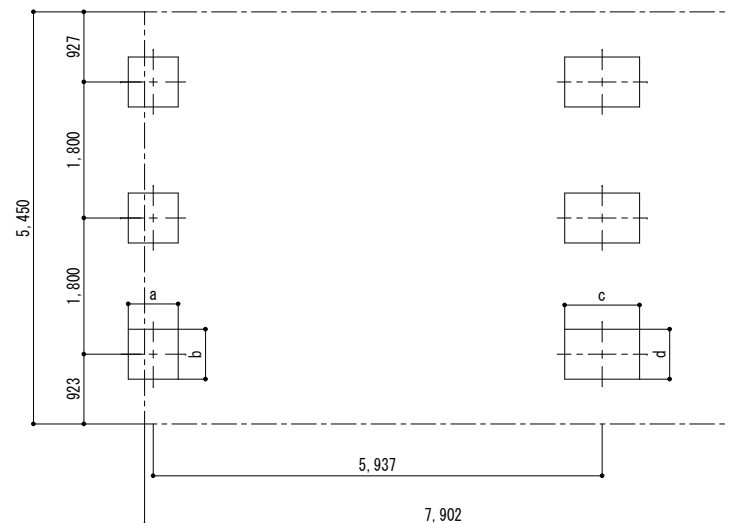
■ 基礎配置図
